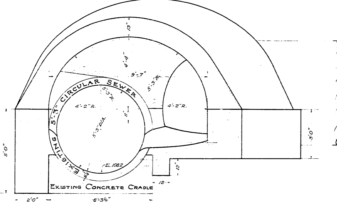
SECTION B-B Scale: 1/2"=1'-0"
