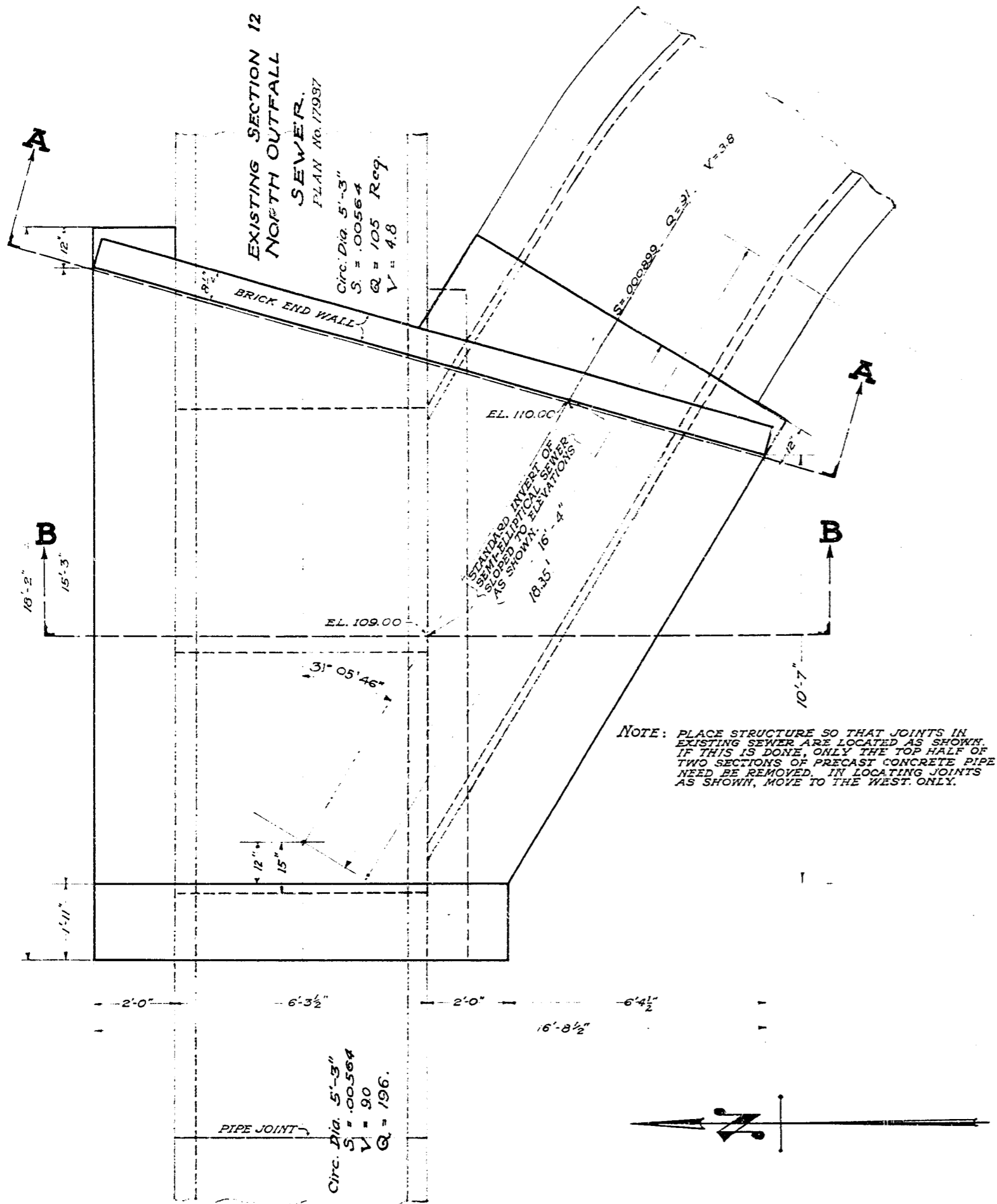
PLAN Scale: 1/2"=1'-0"
